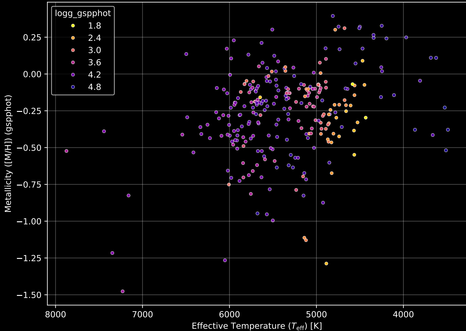
APOGEE DR17 Field: [256+26] Stellar Population Parameters (n= 272)
